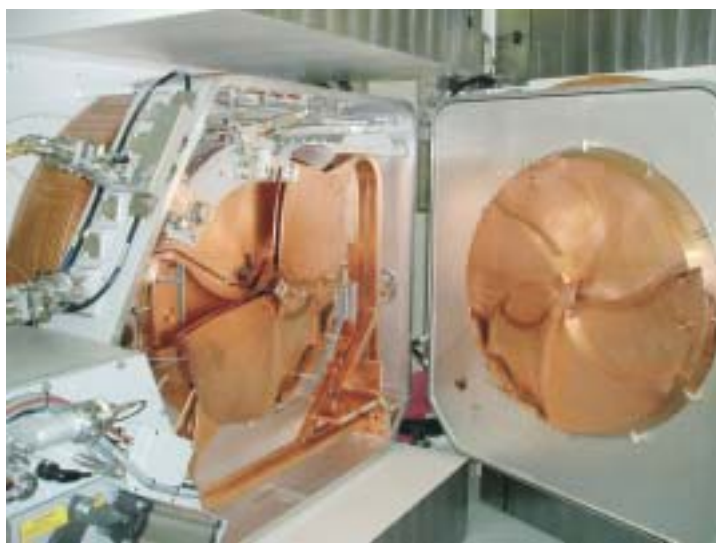
Cyclotron 18 MeV pour la production de Fluor 18. La vue de l'appareil ouvert montre les quadrupoles permettant l'accélération des protons (équipement General Electric).
