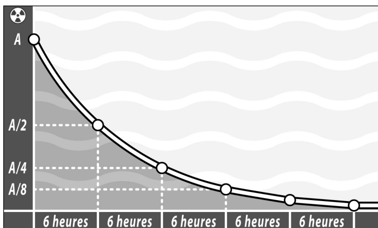
Figure 3. Décroissance et demi-vie : une substance radioactive perd la moitié de son activité ( A ) ou bout d'une période (ou demi-vie) suivant une courbe de décroissance régulière. La décroissance du Technétium 99m de période 6 heures est donnée à titre d'exemple.
