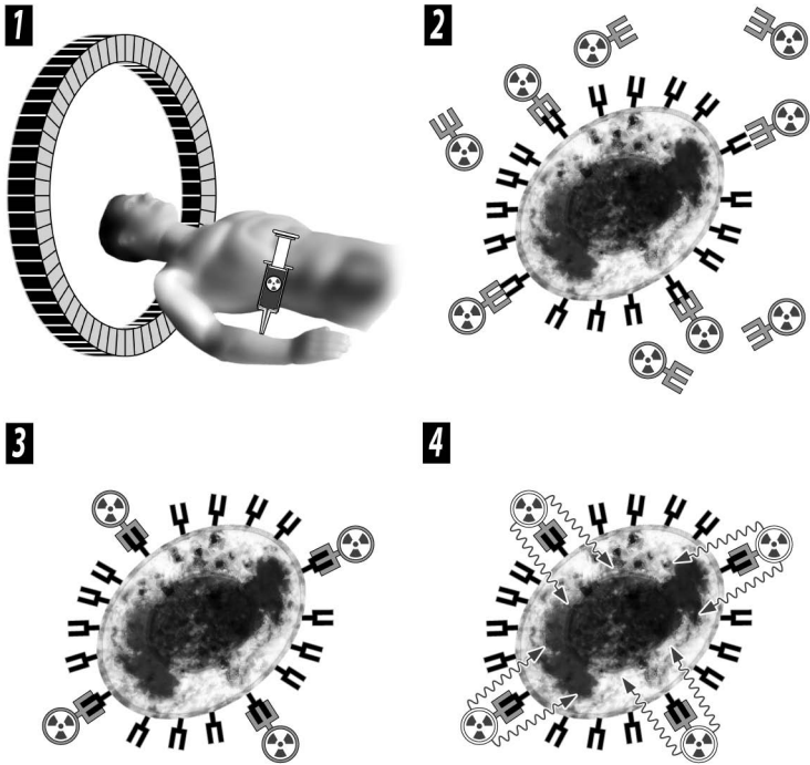
Figure 10. Principe de la radiothérapie métabolique: la substance radioactive fixée à un vecteur est injectée au patient (1). La cellule cancéreuse possède en surface des récepteurs spécifiques que le vecteur est capable de reconnaître. Ce vecteur se fixe sur ces récepteurs qui n'existent qu'en grand nombre sur les cellules tumorales (2). Pendant que les molécules qui n'ont pas trouvé à s'accoupler s'éliminent de façon naturelle du corps (3), les radionucléides se désintègrent lentement en détruisant les cellules de leur environnement direct (4) par émission bêta.
