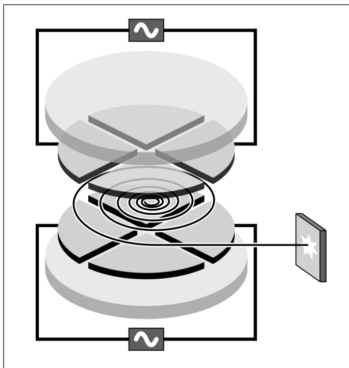
Figure 13. Schéma de principe du fonctionnement d'un cyclotron: des protons générés au centre du cyclotron sont accélérés dans une enceinte placée sous vide au moyen d'un champ électromagnétique symbolisé par les quatre quadrans. Quand leur vitesse idéale est atteinte, les protons sont projetés sur une cible externe qui contient l'élément à transformer. La réaction de transformation nucléaire, donc de production du radionucléide, a lieu dans cette cible. En fin de production, le radionucléide formé sera isolé et purifié dans une cellule de radiochimie externe au cyclotron.
